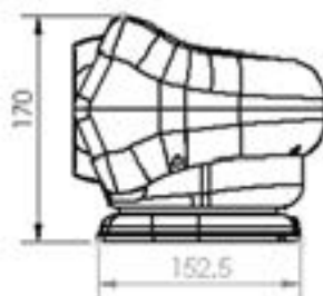
GOL000005 (12 V)
